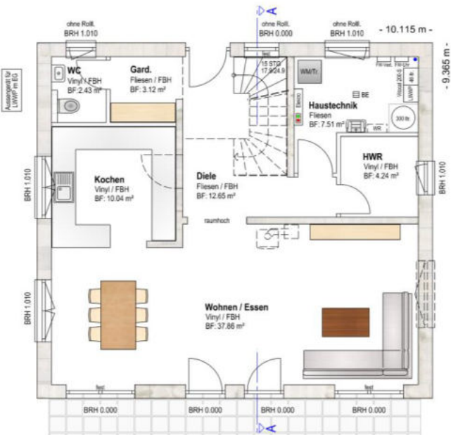
GRUNDRISS ERDGESCHOSS - ohne Keller
