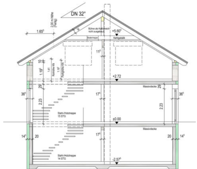
QUERSCHNITT A-A - mit Keller
