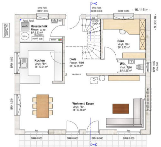
GRUNDRISS ERDGESCHOSS, Variante 1 - ohne Keller
