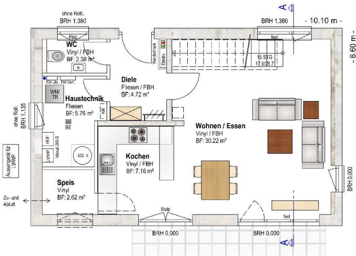
GRUNDRISS ERDGESCHOSS - ohne Keller
