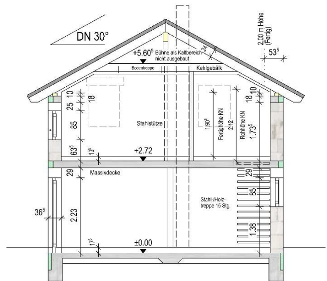
QUERSCHNITT A-A - ohne Keller
