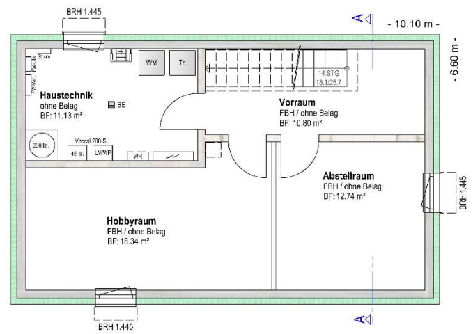
GRUNDRISS UNTERGESCHOSS
